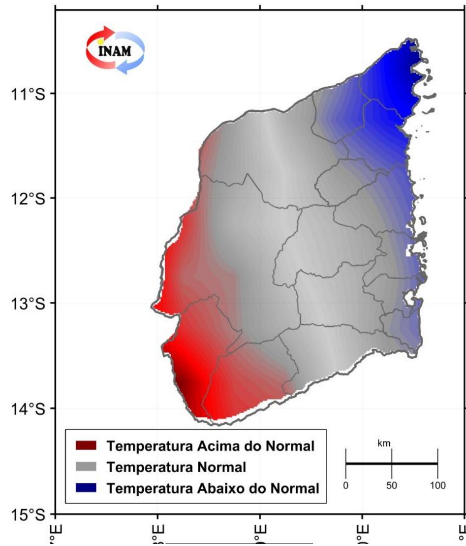
Previsão Climática da Temperatura Máxima: FMA 2022
