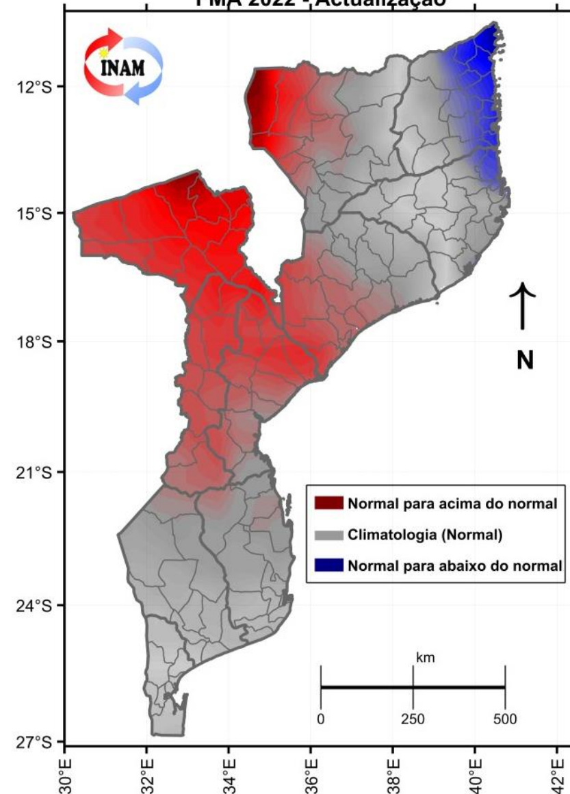
Previsão Climática da Temperatura Máxima: FMA 2022 - Atualização
