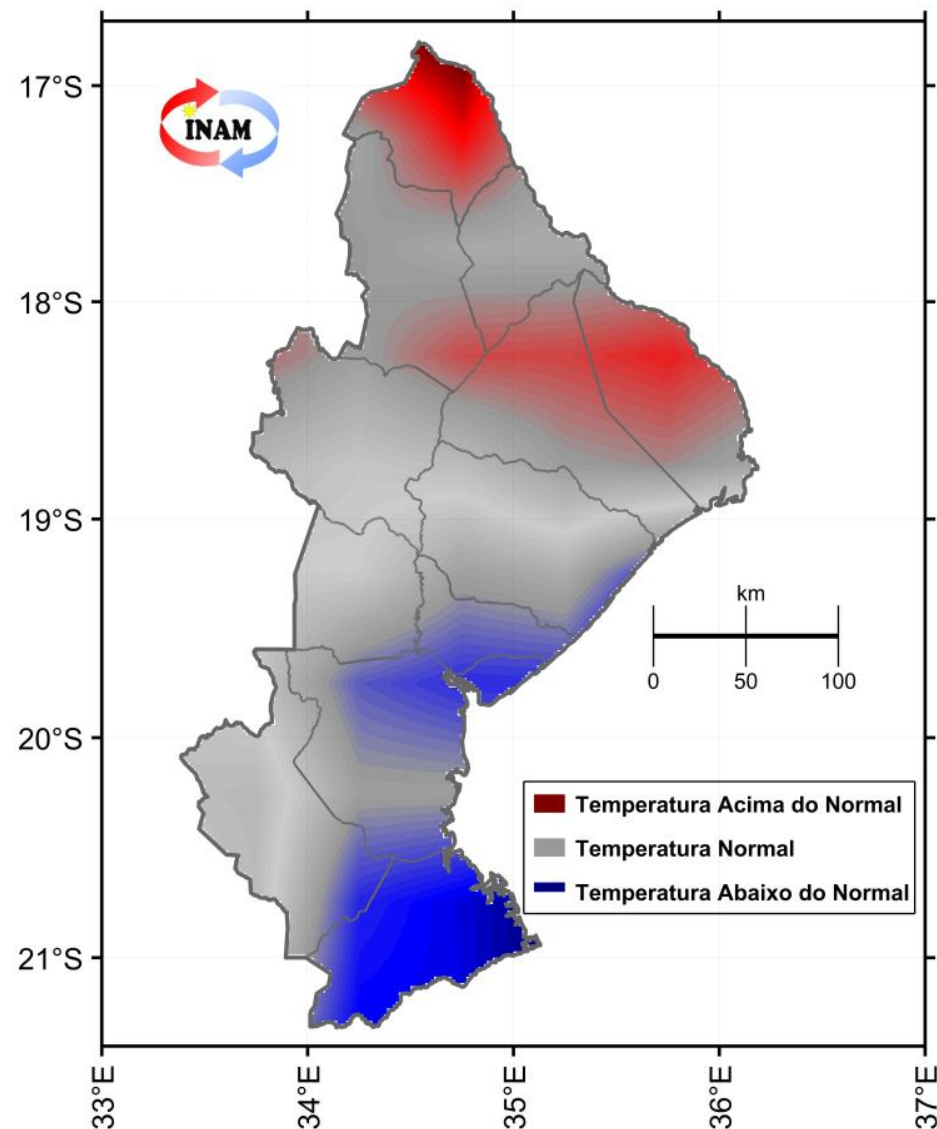
Previsão Climática da Temperatura Máxima: FMA 2022
