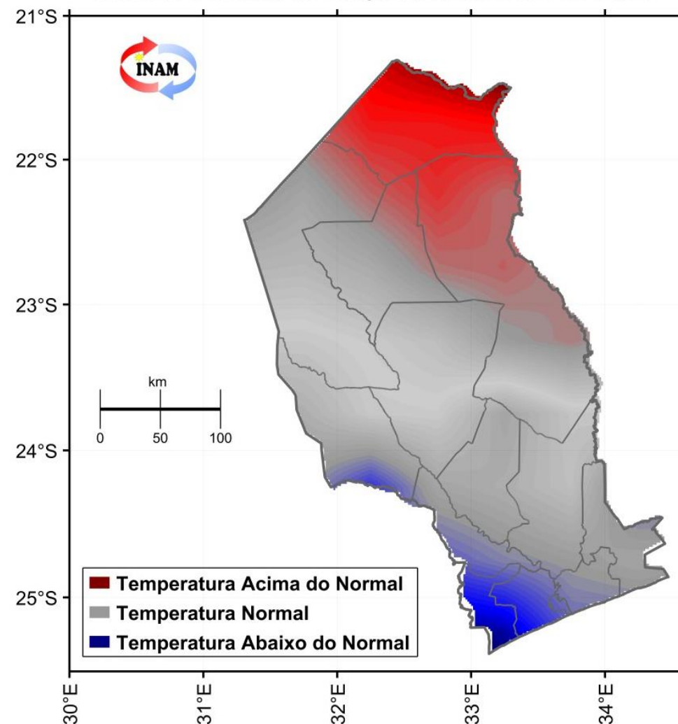
Previsão Climática da Temperatura Máxima: FMA 2022
