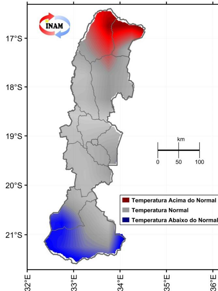
Previsão Climática da Temperatura Máxima: FMA 2022
