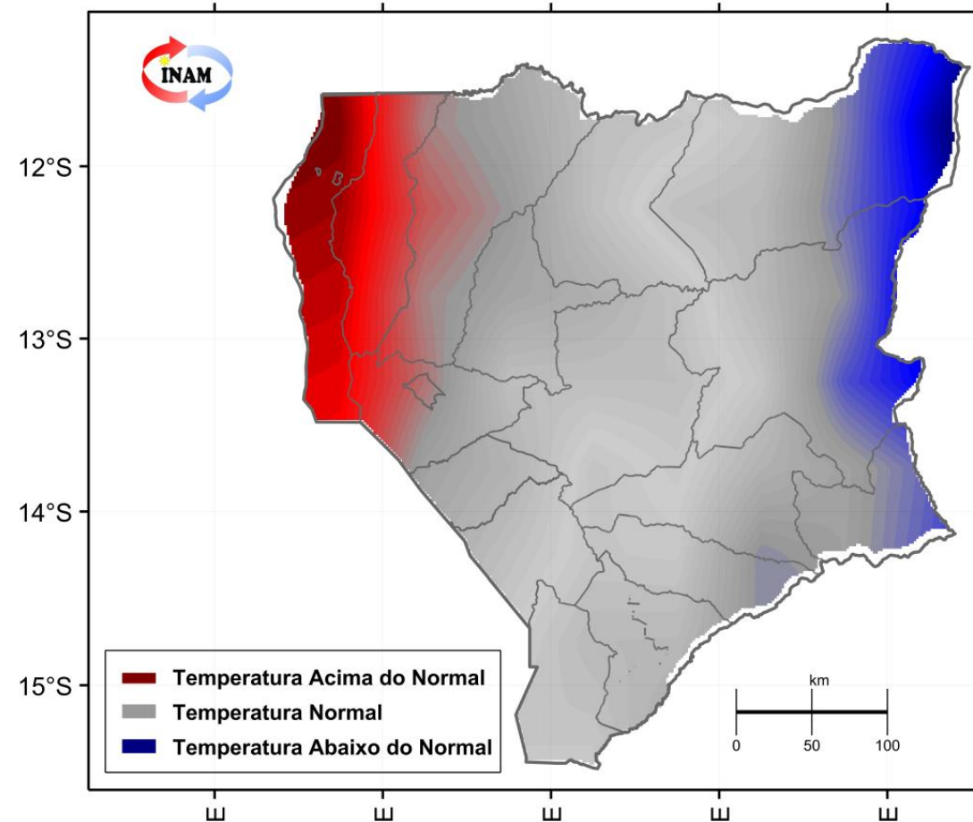
Previsão Climática da Temperatura Máxima: FMA 2022
